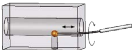
Kugelpkopfform: Entfernt nur die Grate der Querbohrung ohne die Bohrungswandung zu beschädigen.
