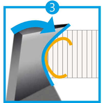
Schließlich wird der Span im Zentrum der Fase vom Werkstück abgeschert. Erst dann verlässt das Werkzeug das Werkstück.
