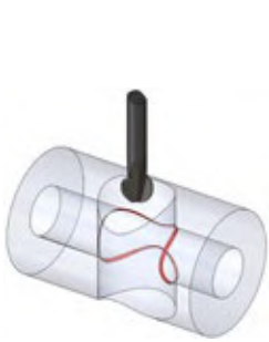
UNTERBROCHENE BOHRUNG ACHSVERSETZT Querbohrung > Hauptbohrung
