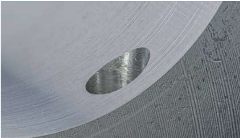
OBN: Achsversetzter Bohrungsaustritt in die Querbohrung in einem Alu-Bauteil. Mit dem ExBurrDrill ist selbst bei dieser Bearbeitung fast kein Grat zu messen.
